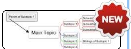
Freeplane p.22
